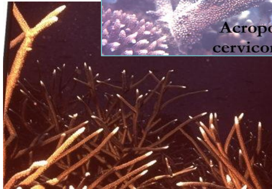
Polypiers coloniaux actuels ou coraux 1: Madrépore; squelette calcaire; chaque petit « trou » correspond à un organisme ou polype 2: Acropores avec squelette et polypes vivants; 2a: milieu moyennement agité; 2b: milieu calme
