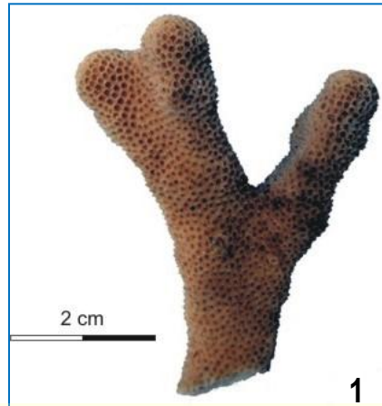
Polypiers coloniaux actuels ou coraux 1: Madrépore; squelette calcaire; chaque petit « trou » correspond à un organisme ou polype 2: Acropores avec squelette et polypes vivants; 2a: milieu moyennement agité; 2b: milieu calme
